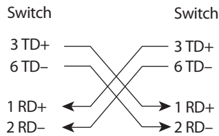
Figura 61 - Esquema de cable de tipo cruzado con dos cables trenzados
