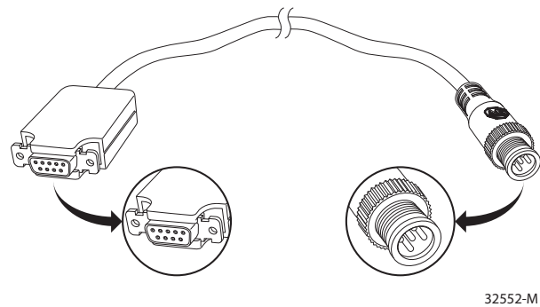
Figura 52 - Configuración de pines del puerto de consola
