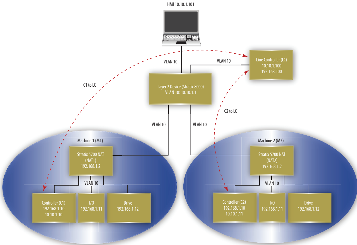
Figura 10 - Ejemplo de capa 2
