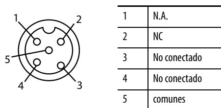
Figura 55 - Ejemplo de cableado de entradas y salidas de alarmas
