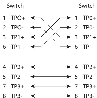
Figura 50 - Esquema de cable de tipo cruzado con cuatro cables trenzados
