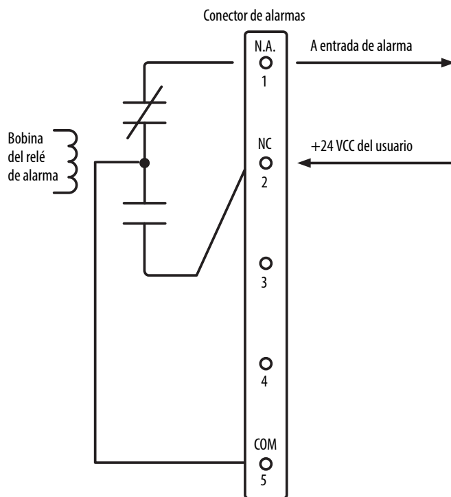
Figura 55 - Ejemplo de cableado de entradas y salidas de alarmas
