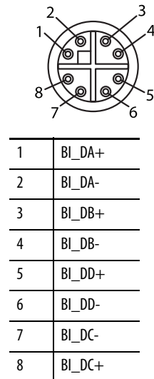
Figura 46 - Configuraciones de pines del conector 100/1000
