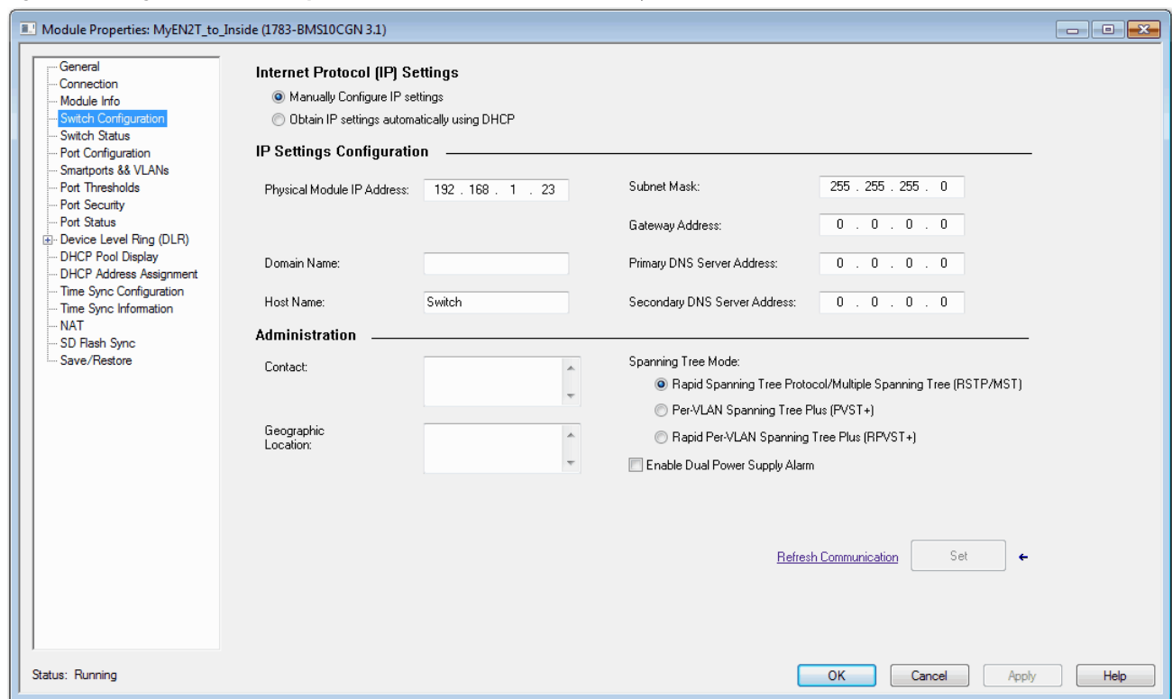
Figura 27 - Configuración del switch para switches Stratix 5400, Stratix 5700 y ArmorStratix 5700
