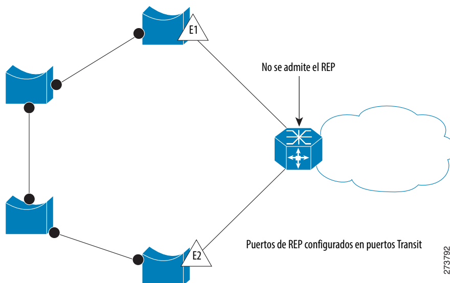
Figura 23 - Ejemplo de topología de anillo
