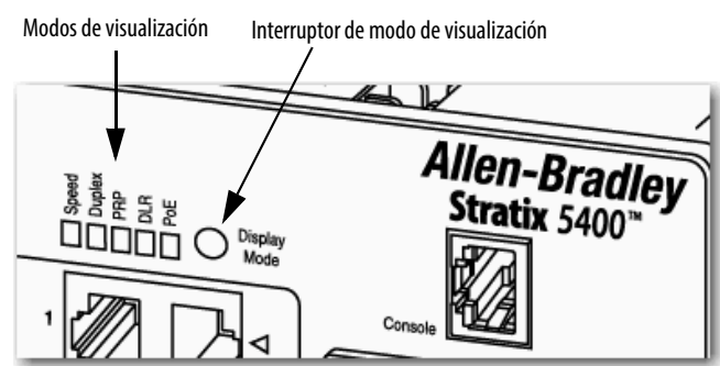
Figura 34 - Interruptor de modo de visualización de Stratix 5400
