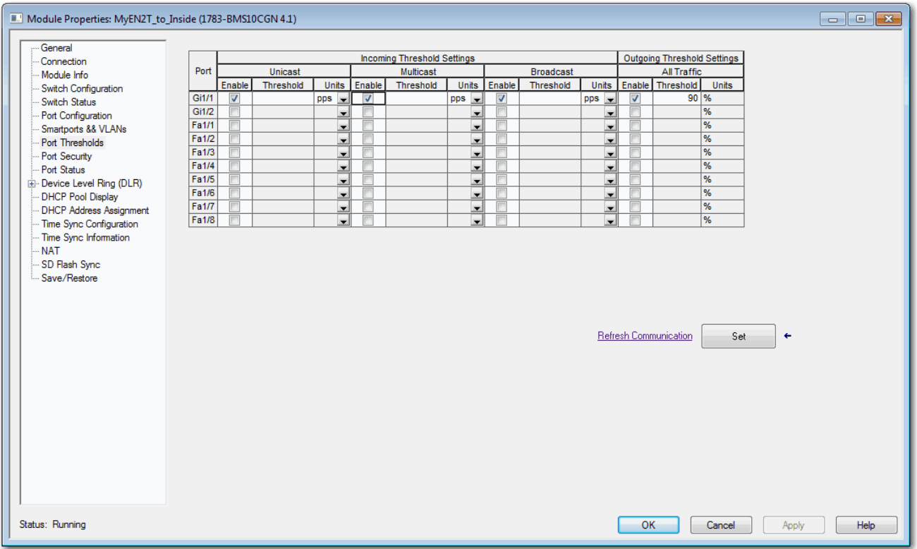
Figura 15 - Umbrales de puertos para switches Stratix 5400, Stratix 5700 y ArmorStratix 5700
