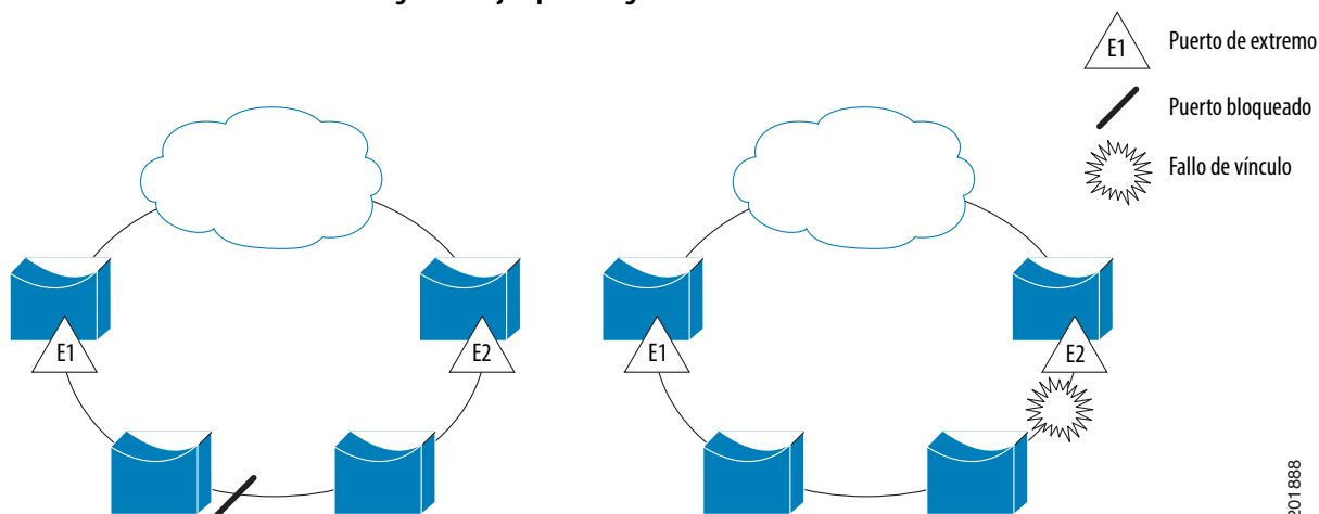
Figura 21 - Ejemplo de segmento abierto
