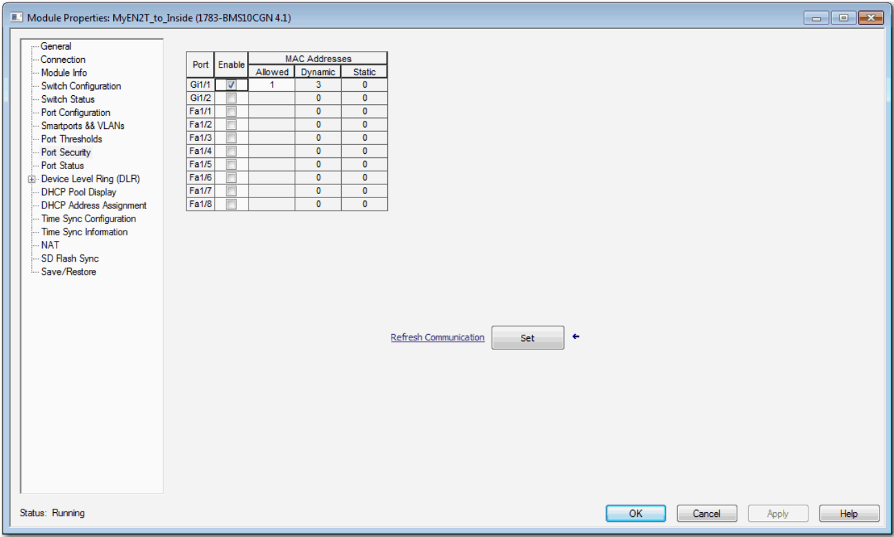
Figura 12 - Seguridad de puertos de switches Stratix 5400, Stratix 5700 y ArmorStratix 5700
