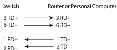
Figura 39 - Esquema de cable de tipo directo con dos cables trenzados
