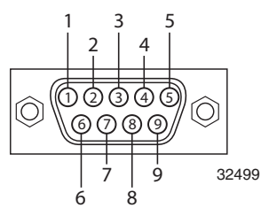
Figura 53 - Configuración de pines del conector DB-9
