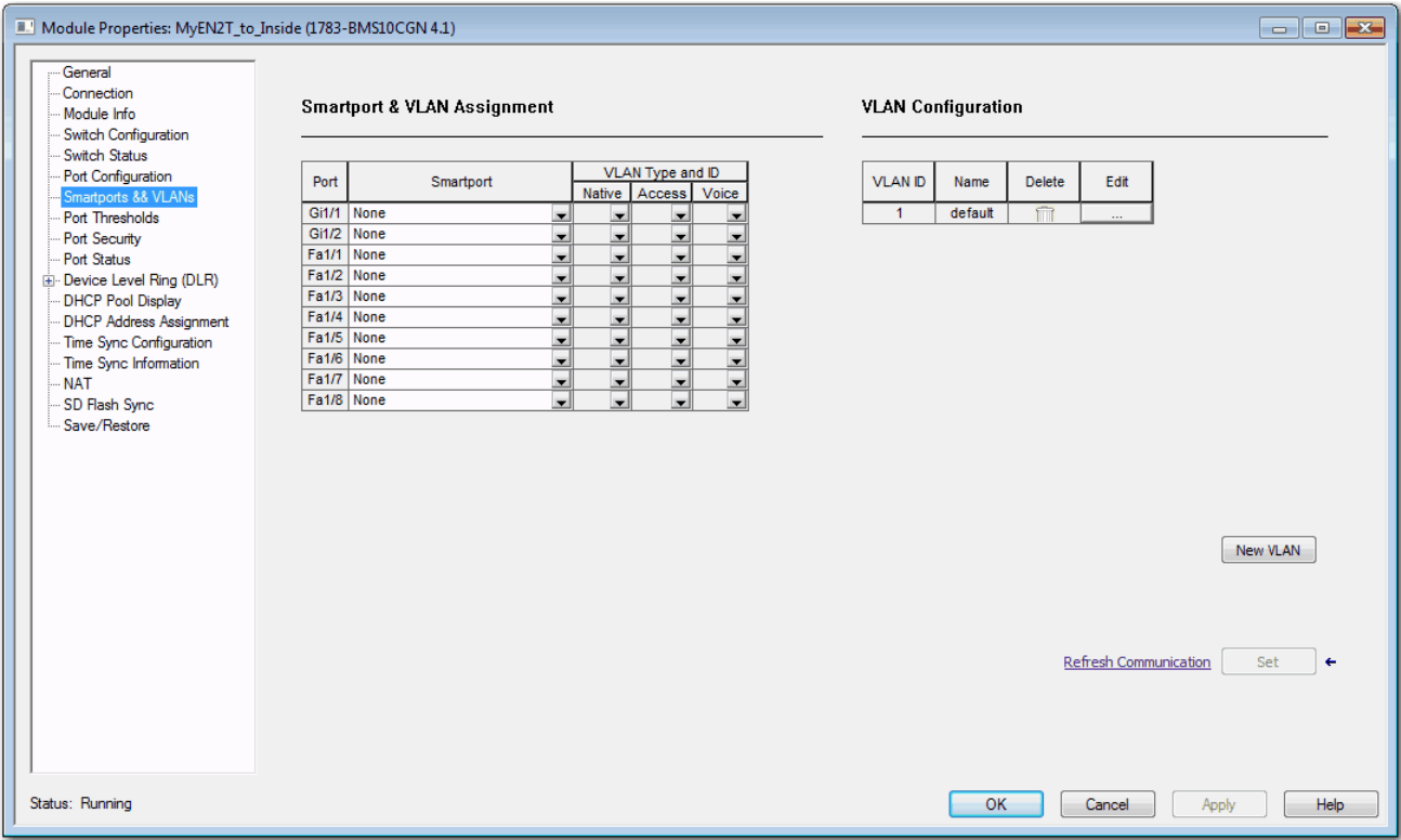
Figura 29 - Configuración de VLAN para switches Stratix 5400, Stratix 5700 y ArmorStratix 5700
