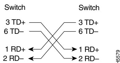
Figura 50 - Esquema de cable de tipo cruzado con cuatro cables trenzados
