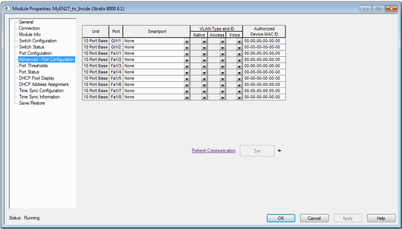
Figura 13 - Configuración avanzada de puertos de switches Stratix 8000/8300
