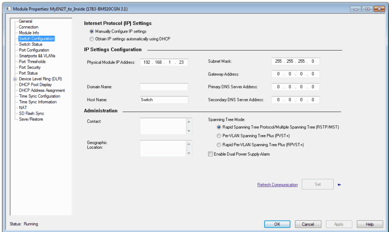
Figura 1 - Configuración del switch en switches Stratix 5700 y ArmorStratix 5700
