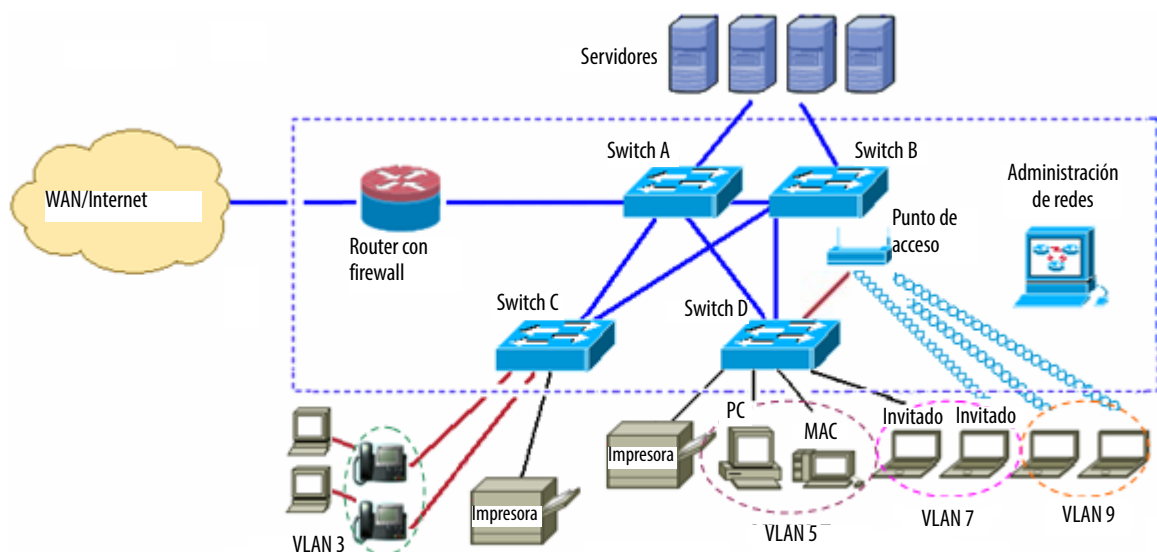
Figura 28 - Ejemplo de VLAN
