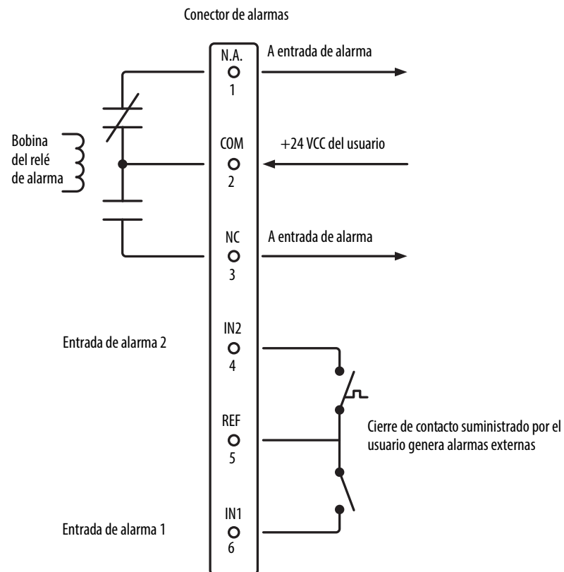
Figura 44 - Ejemplo de cableado de entradas y salidas de alarmas
