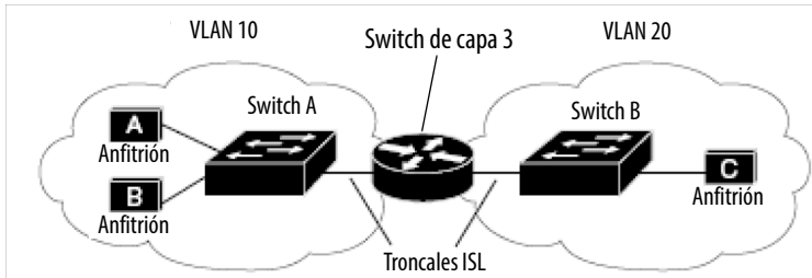
Figura 24 - Ejemplo de topología de encaminamiento
