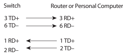
Figura 48 - Esquema de cable de tipo directo con dos cables trenzados
