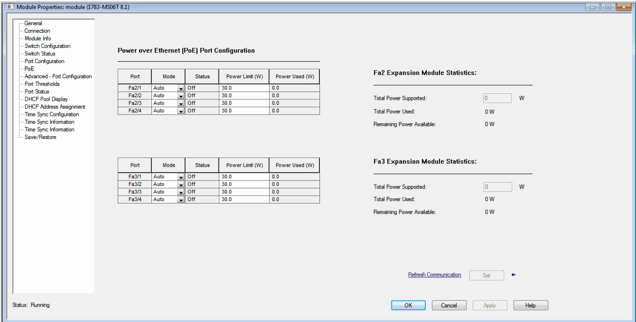
Figura 20 - Configuración PoE para switches Stratix 8000/8300
