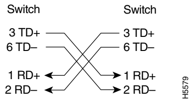
Figura 42 - Esquema de cable de tipo cruzado con cuatro cables trenzados
