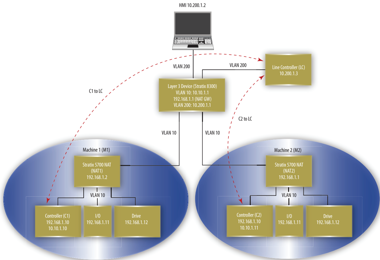
Figura 9 - Ejemplo de capa 3
