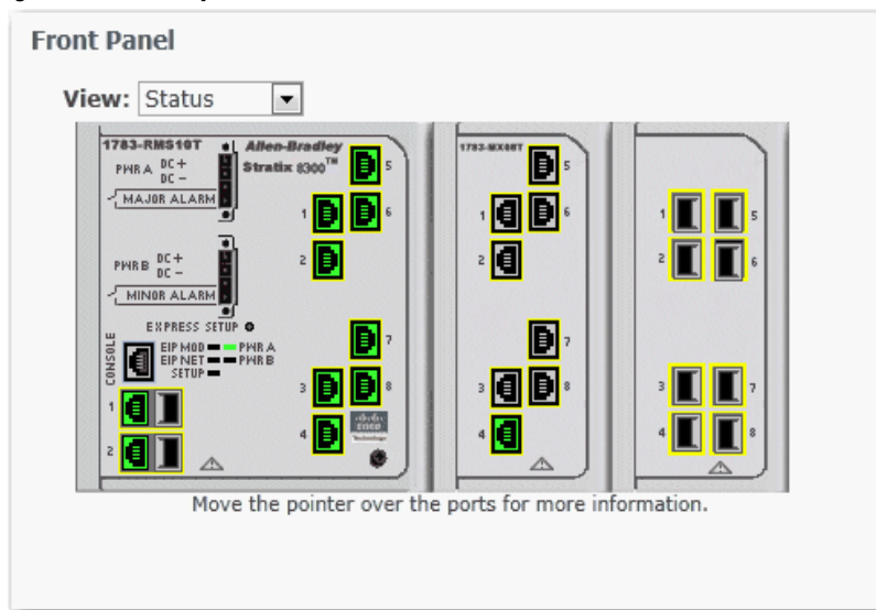
Figura 35 - Vista del panel frontal de Stratix 8000/8300
