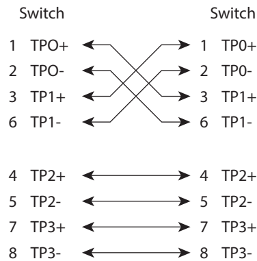
Figura 62 - Esquema de cable de tipo cruzado con cuatro cables trenzados
