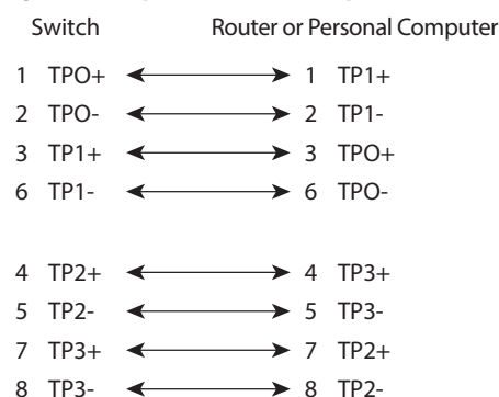
Figura 60 - Esquema de cable de tipo directo con dos cables trenzados
