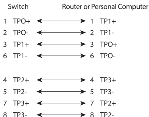
Figura 40 - Esquema de cable de tipo directo con dos cables trenzados
