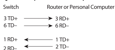
Figura 59 - Esquema de cable de tipo directo con dos cables trenzados
