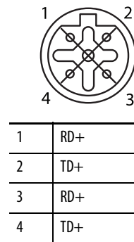
Figura 45 - Configuraciones de pines del conector 10/100
