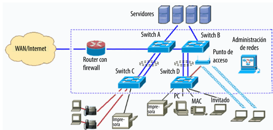
Figura 8 - Ejemplo de EtherChannel
