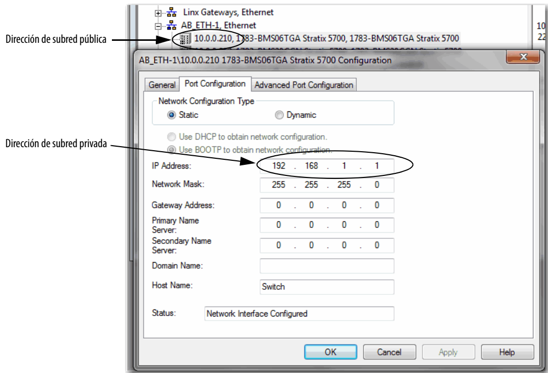
Figura 11 - Direcciones de subredes públicas y privadas en el software RSLinx
