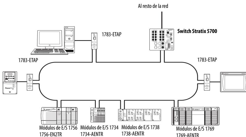
Figura 7 - Ejemplo de topología de anillo a nivel de dispositivos
