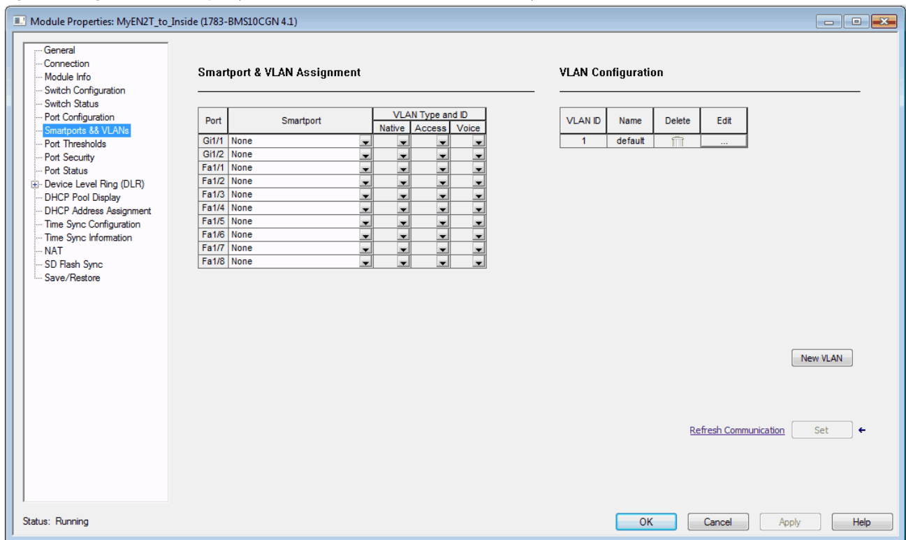
Figura 25 - Asignación de Smartport y VLAN en switches Stratix 5400, Stratix 5700 y ArmorStratix 5700
