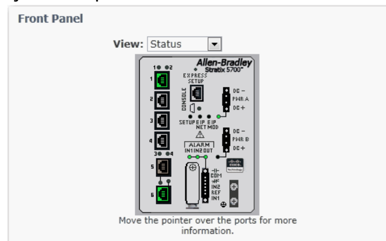
Figura 32 - Vista del panel frontal de Stratix 5700
