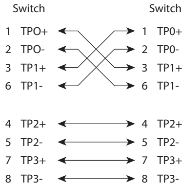
Figura 42 - Esquema de cable de tipo cruzado con cuatro cables trenzados
